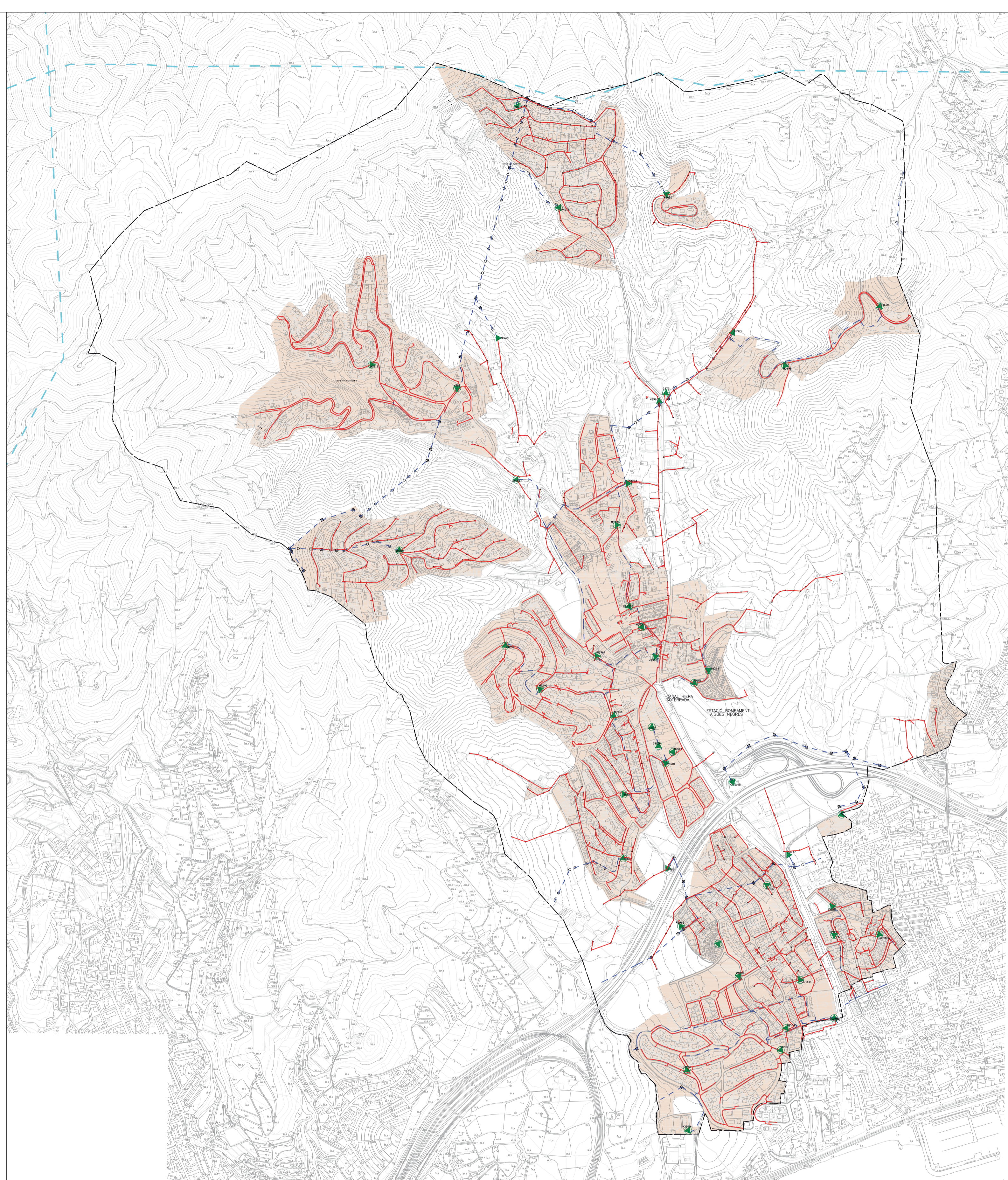
XARXA D'ELECTRICITAT
